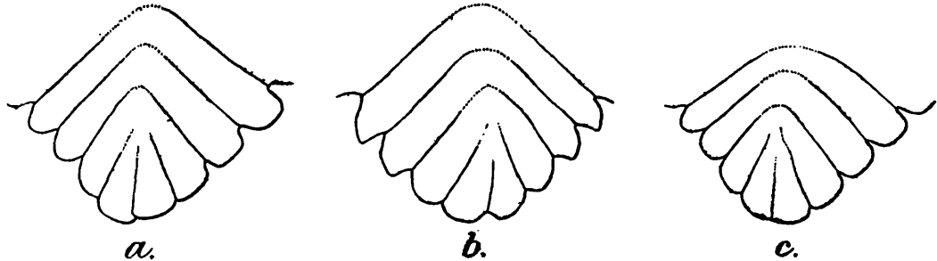
TEXT-FIG. 19.— Palaegyge pica , sp. nov.
