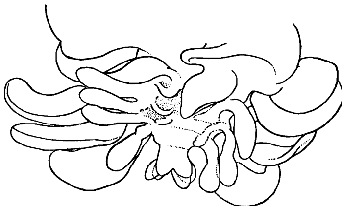
TEXT-FIG. 3.— Hemiarthrus sp.
